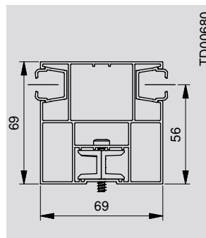
Guida doppia 69 x 69 mm
