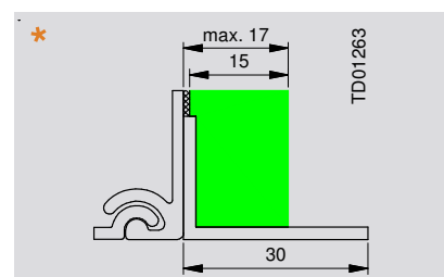
Pannello styrodur 15 mm
