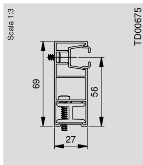
Guida stretta 27 x 69 mm
