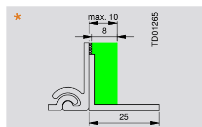
Pannello styrodur 8 mm Altre opzioni per INTEGO v. „Optional frangisole“ pagina 174
