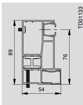
Optional guida distanziata 54 x 89 mm
