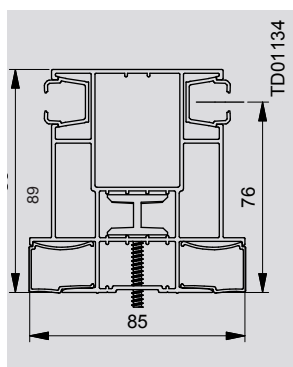
Optional guida doppia distanziata 85 x 89 mm
