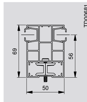
Optional guida doppia stretta 50 x 69 mm
