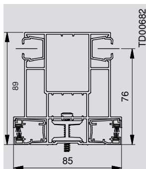
Guida doppia 85 x 89 mm
