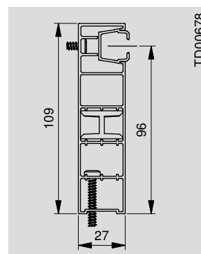
Guida singola 27 x 109 mm (con isolamento posteriore da 40 mm)
