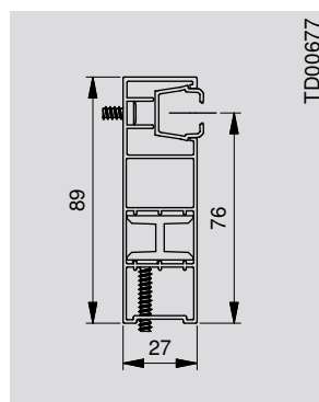
Guida singola 27 x 89 mm (con isolamento posteriore 20 mm)
