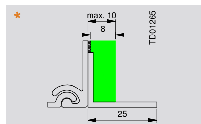
Pannello styrodur 8 mm
